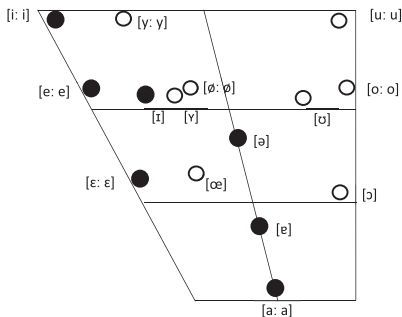
orale Monophthonge
