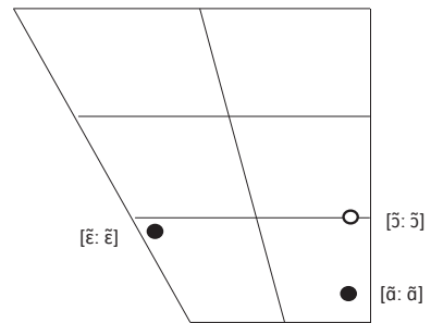
nasalisierte Monophthonge
